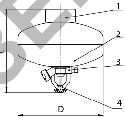
Рисунок 1 – Устройство модулей МПП «МИГ» 1 – подвеска, 2 – корпус, 3 – запорно-пусковое устройство, 4 – тепловой замок.
