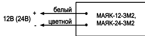
Рис. 1. Схема подключения
