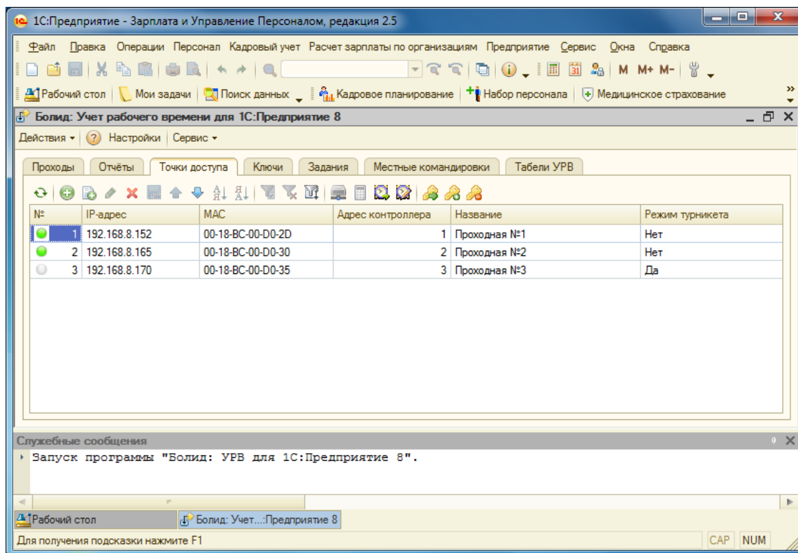
Рисунок 11. Страница «Точки доступа».
