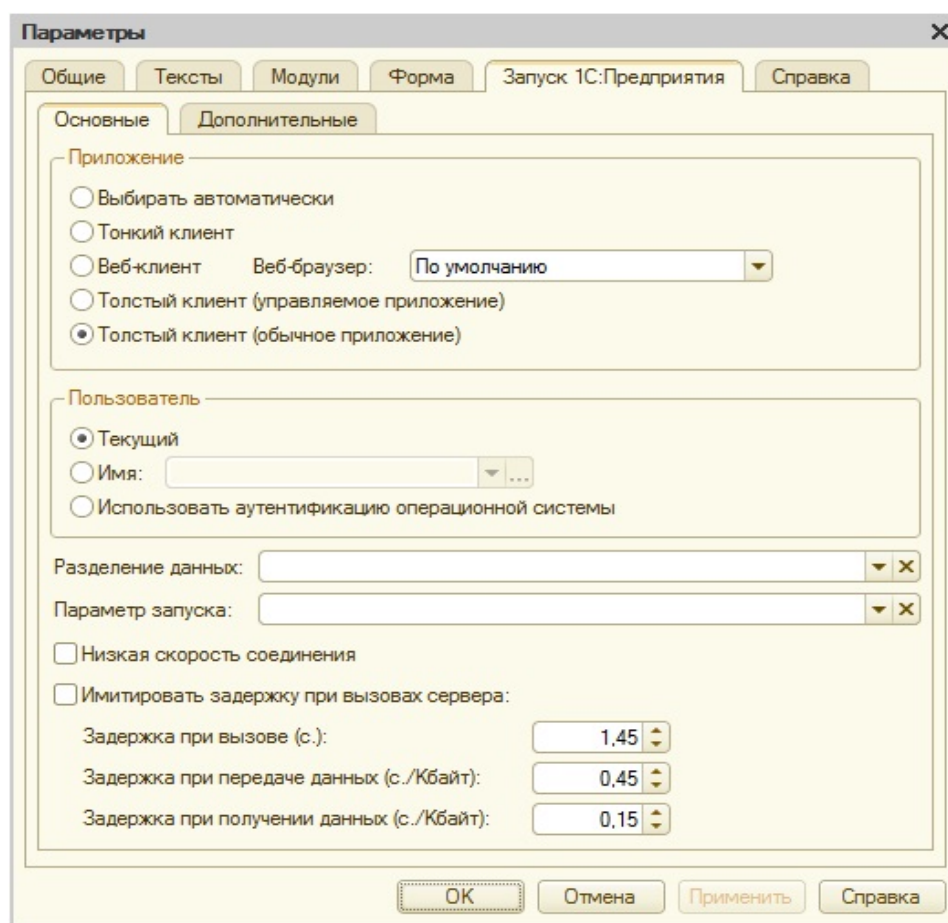
Рисунок 2. Параметры настройки «1С: Предприятие 8», страница «Запуск 1С: Предприятия».
