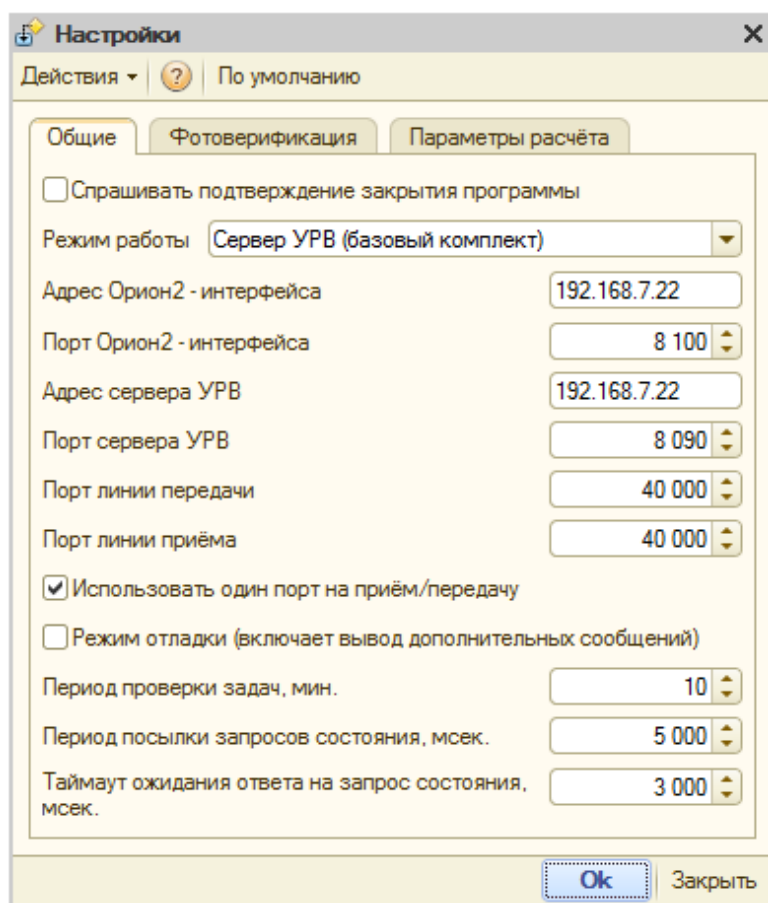
Рисунок 25. Настройки компьютера «Сервер УРВ».
